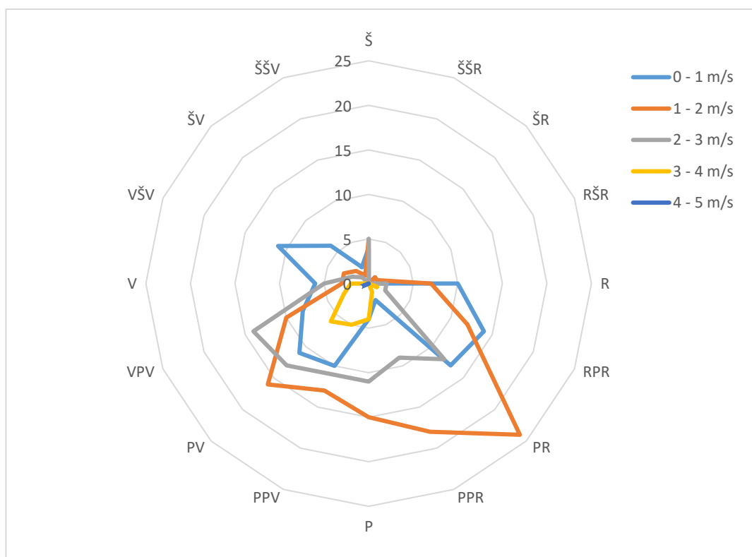
2 pav. Vėjo greitis ir kryptis tyrimo metu
