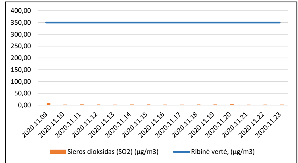
4 pav. Maksimali 1 val. vidurčio sieros dioksido koncentracija tyrimų metu
