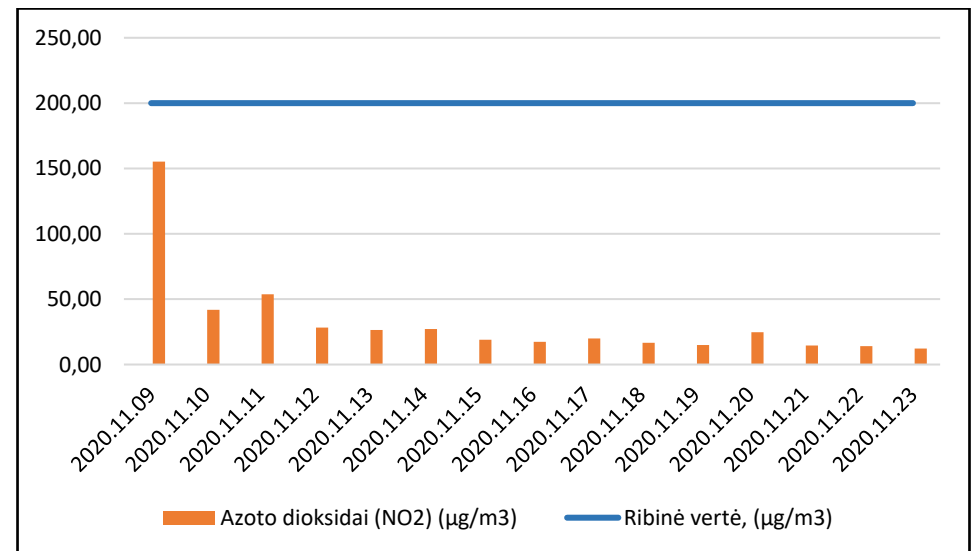
6 pav. Maksimali 1 val. vidurčio azoto dioksido koncentracija tyrimų metu
